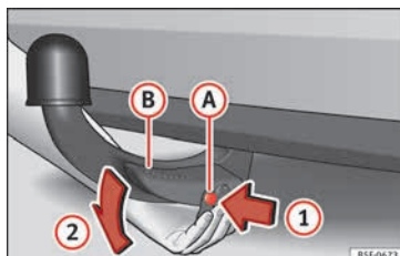
Fig. 229 Soltar la bola desmontable
