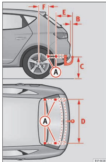
Fig. 232 Puntos de fijación del dispositivo de remolque.
