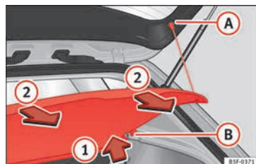
Fig. 159 Portón del maletero abierto con la bandeja del maletero.
