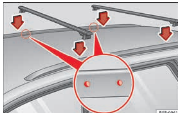
Fig. 183 Leon ST: puntos de fijación de las barras transversales para el portaequipajes del techo.
