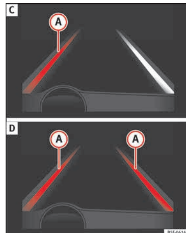
Fig. 207 En la pantalla del cuadro de instrumentos: indicación en la pantalla del sistema de aviso de salida del carril (ejemplo 2).
