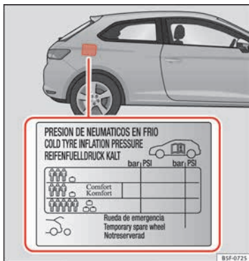
Fig. 237 Ubicación del adhesivo de la presión de inflado de los neumáticos.
