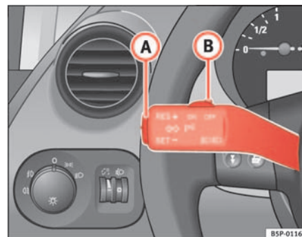
Fig. 143 Palanca de intermitentes y de luz de carretera: mando y tecla basculante para el regulador de velocidad
