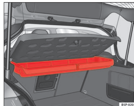
Fig. 117 Alojamiento para el triángulo de preseñalización bajo la bandeja posterior
