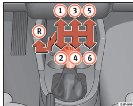
Fig. 132 Detalle de la consola central: esquema de un cambio manual de 6 marchas
