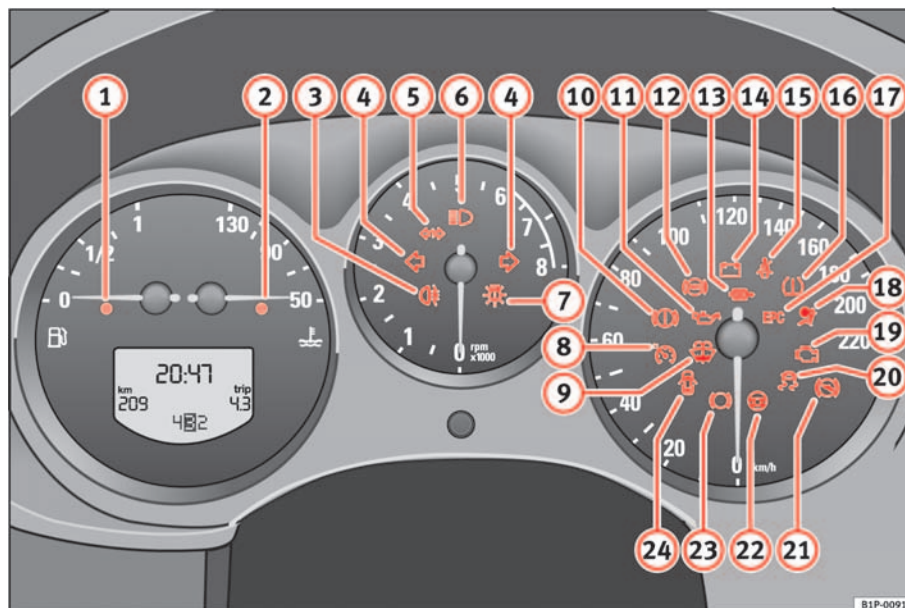
Fig. 47 Testigos de control y de advertencia del cuadro de instrumentos. Algunos de estos testigos pertenecen sólo a determinadas versiones del modelo o forman parte de equipamientos opcionales.
