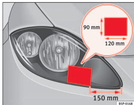
Fig. 144 Faro derecho
