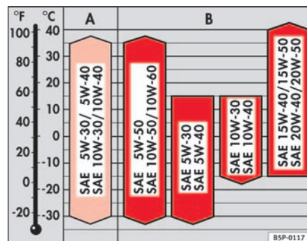
Fig. 153 Tipos de aceite de acuerdo a la temperatura
