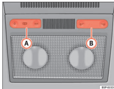
Fig. 81 Revestimiento interior del techo: luces delanteras de lectura tipo 1
