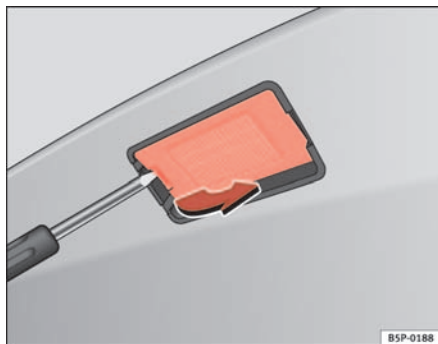
Fig. 190 Luz matrícula
