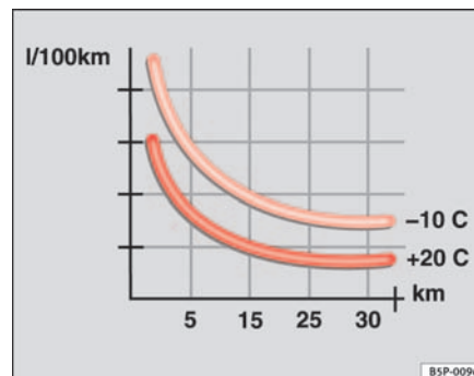
Fig. 148 Consumo de combustible (l/100 km) a dos temperaturas ambiente
