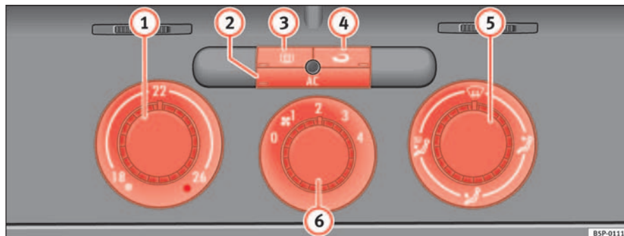
Fig. 124 Mandos del Climatic en el tablero de instrumentos
