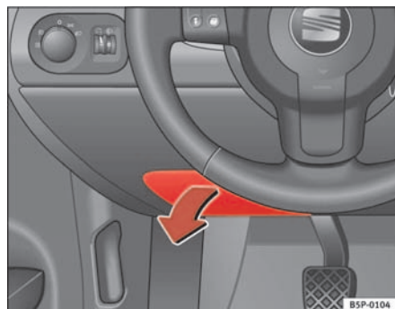
Fig. 171 Tapa de la caja de fusibles en el lado izquierdo del tablero de instrumentos
