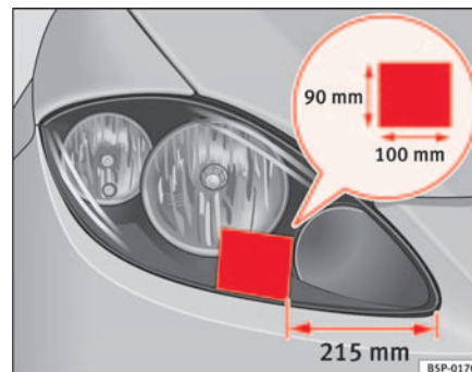
Fig. 146 Faro derecho
