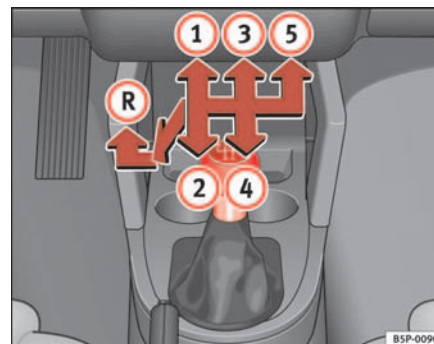
Fig. 131 Detalle de la consola central: esquema de un cambio manual de 5 marchas
