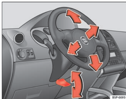
Fig. 127 Ajuste de la posición del volante
