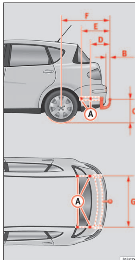
Fig. 149 Puntos de fijación del dispositivo de remolque
