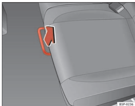
Fig. 96 Barra de desbloqueo del asiento posterior
