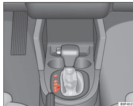
Fig. 133 Consola central: palanca selectora del cambio automático / cambio automático DSG
