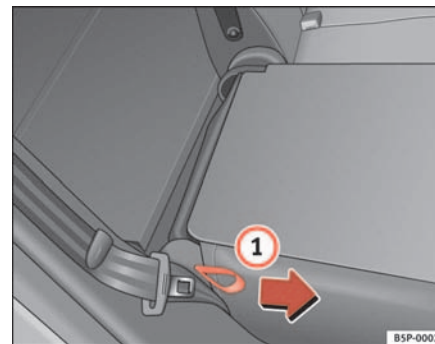
Fig. 99 Abatir o levantar el respaldo del asiento posterior
