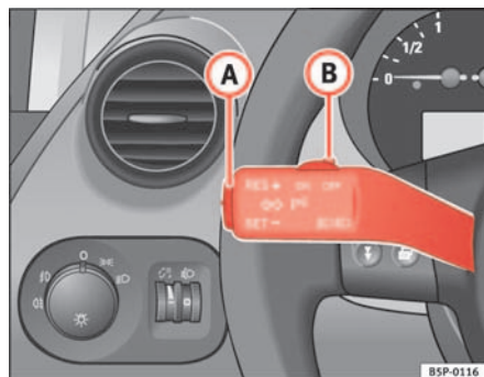
Fig. 142 Palanca de intermitentes y de luz de carretera: mando y tecla basculante para el regulador de velocidad
