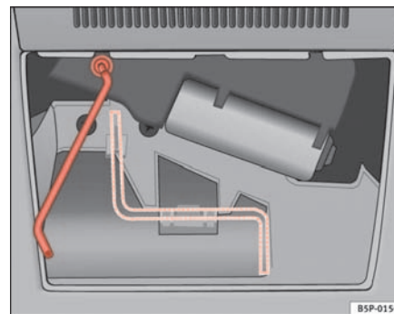
Fig. 73 Manivela cierre de emergencia
