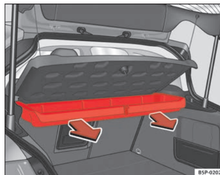
Fig. 124 Desmontaje caja portaobjetos
