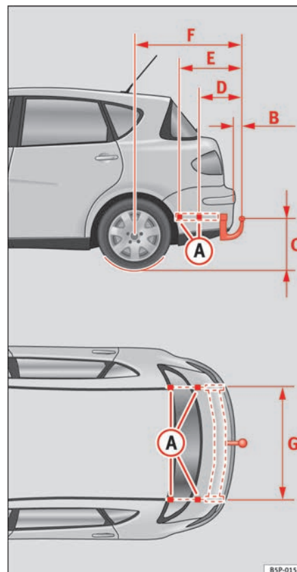
Fig. 151 Puntos de fijación del dispositivo de remolque
