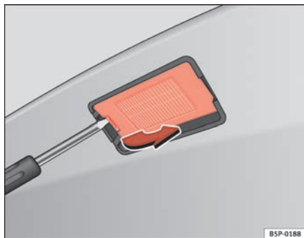
Fig. 193 Luz matrícula
