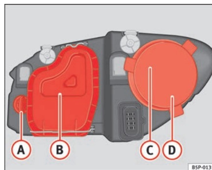
Fig. 176 Lámparas del faro principal
