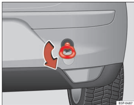
Fig. 199 Atornillado de la argolla de remolque en la parte trasera del vehículo
