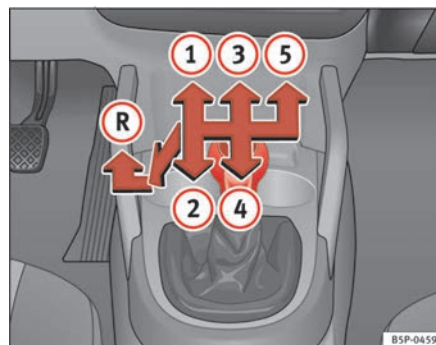
Fig. 137 Detalle de la consola central: esquema de un cambio manual de 5 marchas
