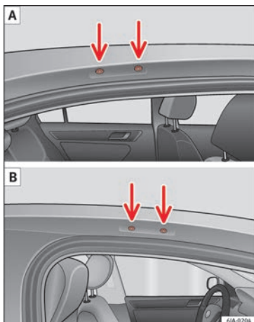
Fig. 168 Puntos de fijación del portaobjetos básico.
