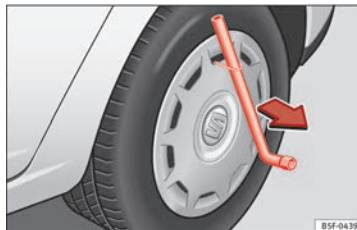
Fig. 60 Retirar el embellecedor integral.
