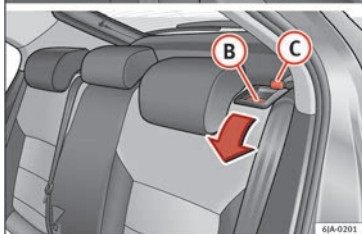
Fig. 148 Desbloqueo del respaldo.
