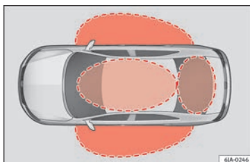
Fig. 124 Sistema de cierre y arranque sin llave Keyless Access: zonas próximas.
