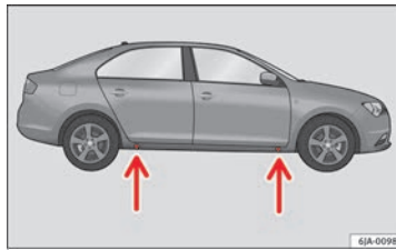
Fig. 64 Cambio de rueda: puntos de apoyo del gato.
