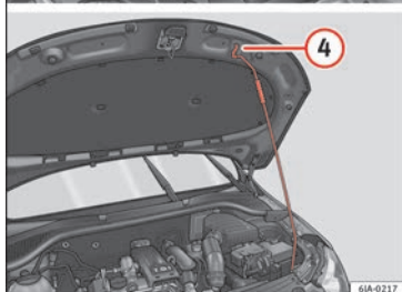
Fig. 204 Bloqueo del capó del vano motor.
