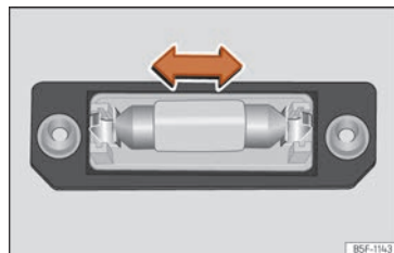
Fig. 109 Cambio de lámpara.
