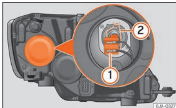
Fig. 93 Cambio de lámpara de la luz de cruce.
