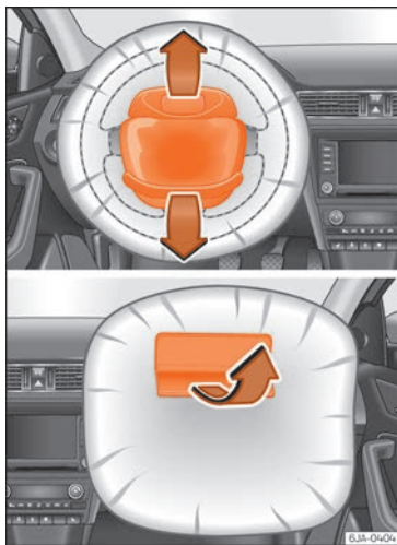
Fig. 19 Cubiertas de los airbags al dispararse los airbags frontales.
