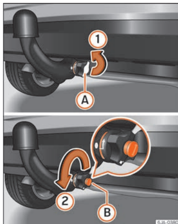
Fig. 239 Quitar la tapa de la cerradura/abrir con llave la cerradura.
