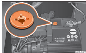
Fig. 249 Batería: indicador de nivel de electrolito.
