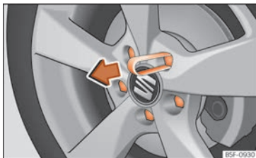
Fig. 61 Retirar la tapa del tornillo de la rueda.
