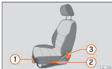
Fig. 12 Asientos delanteros: ajuste manual del asiento.
