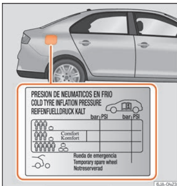
Fig. 251 Ubicación del adhesivo de la presión de inflado de los neumáticos.
