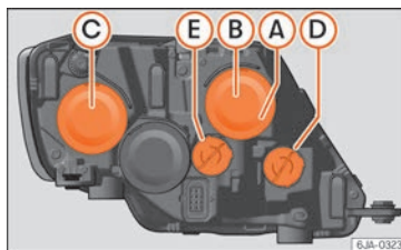
Fig. 89 Lámparas del faro principal.
