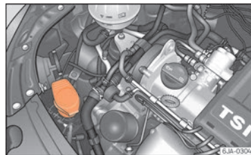
Fig. 247 Vano motor: depósito del sistema lavacristales.
