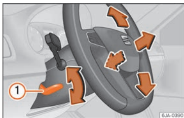
Fig. 17 Palanca en la parte inferior del lateral izquierdo de la columna de dirección.
