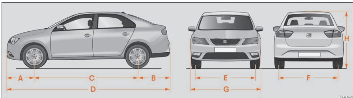
Fig. 255 Dimensiones
