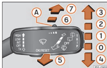
Fig. 35 Manejo del limpiaparabrisas y limpialuneta.
