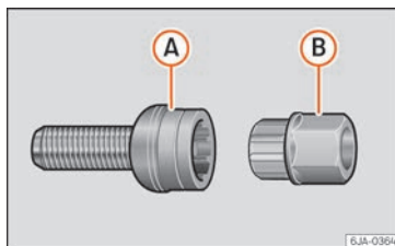
Fig. 62 Tornillo de seguridad para ruedas con adaptador.
