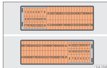
Fig. 86 Vista esquemática de la caja de fusibles a la izquierda/derecha del volante.
