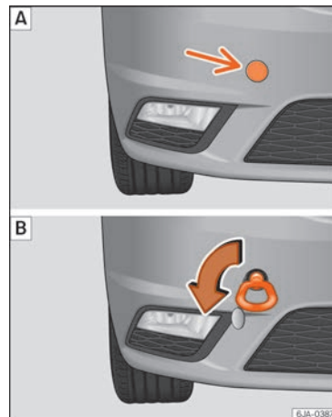
Fig. 66 Parte derecha del parachoques delantero: argolla de remolque enroscada.
