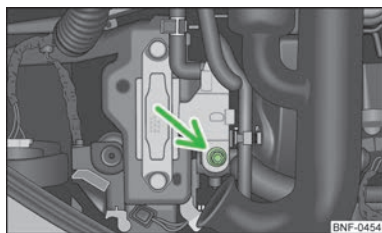
Fig. 117 Vano motor: Paunto de masa del motor
