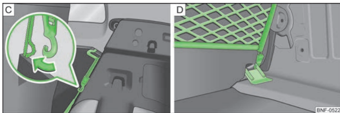
Fig. 42 Redes de retención: Detalle de la sujeción detrás de los asientos posteriores
