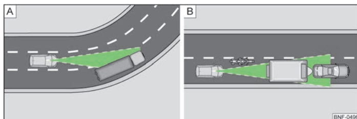
Fig. 72 Vehículo en el área de una curva/Motociclista delantero fuera del radio de acción del sensor láser
