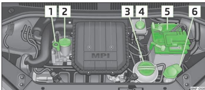
Fig. 99 Motor de gasolina MPI de 1,0 l/55 kW
