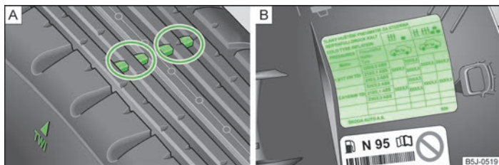
Fig. 105 Perfil de los neumáticos con indicadores de desgaste/tapa del depósito abierta con una tabla de los valores para tamaños de neumáticos y valores de inflado
