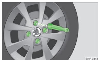
Fig. 111 Cambio de rueda: Aflojar los tornillos de rueda con el mango del destornillador
