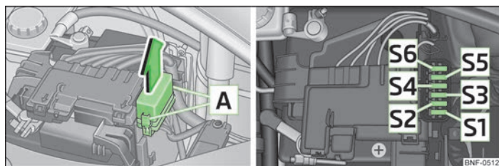
Fig. 120 Vano motor: Tapa de la caja de fusibles/fusibles
