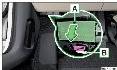
Fig. 167 Retirar la tapa de la caja de fusibles
