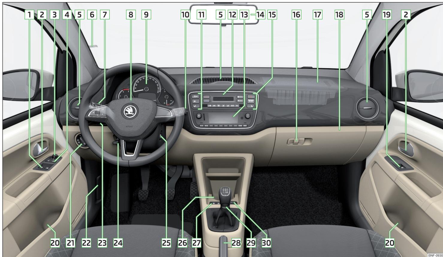
Fig. 17 Ejemplo del puesto de conducción con el volante a la izquierda
