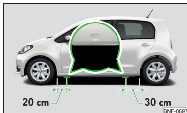
Fig. 154 Travesa de toma para el gato
