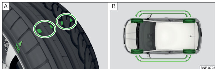
Fig. 146 Indicador de desgaste de los neumáticos / cambio de las ruedas
