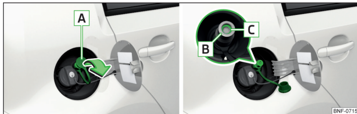
Fig. 136 Tubos de alimentación de gas
