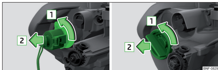
Fig. 175 Cambiar la bombilla para luz intermitente delantera: Variante 1 / Variante 2
