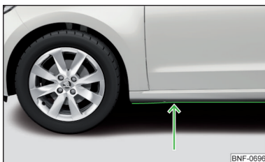
Fig. 127 Altura de agua máxima permitida en vadeos
