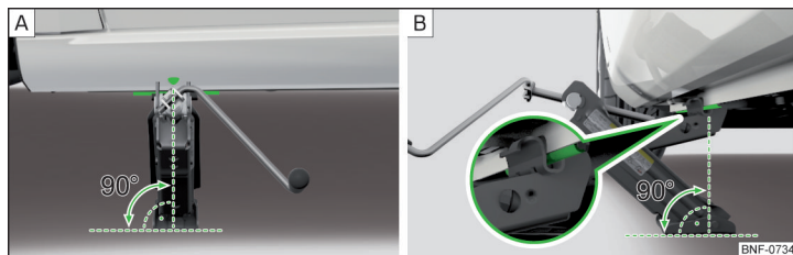
Fig. 155 Colocar el gato
