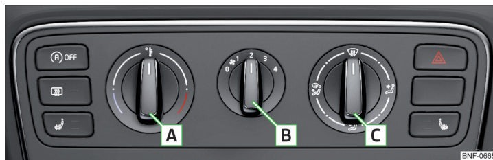
Fig. 88 Elementos de mando de la calefacción
