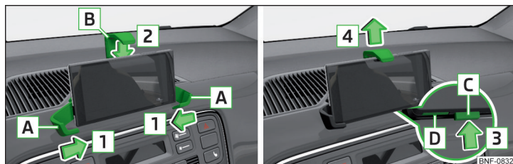
Fig. 79 Colocar el teléfono / Retirar el teléfono
