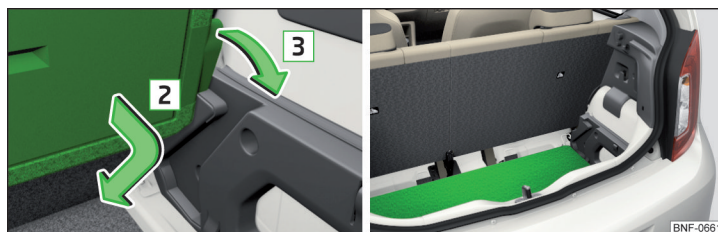
Fig. 85 Piso de carga variable: bajar / en el estado bajado
