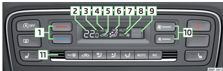
Fig. 90 Elementos de mando del Climatronic
