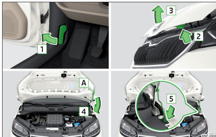
Fig. 138 Abrir el capó
