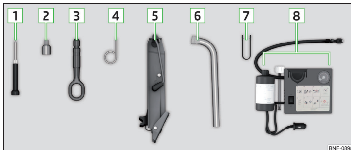
Fig. 149 Equipo de herramientas a bordo
