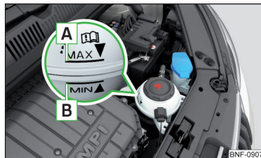
Fig. 142 Depósito de compensación del líquido refrigerante
