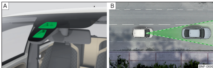
Fig. 131 Sensor láser/zona de detección
