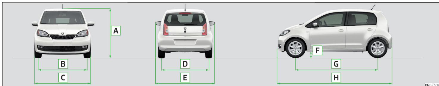
Fig. 182 Dimensiones del vehículo
