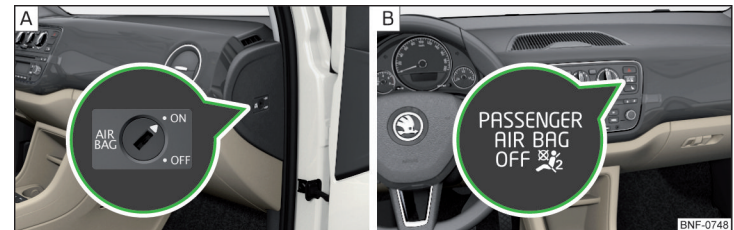
Fig. 11 Conmutador de llave para el airbag lateral del acompañante/Testigo para el airbag delantero del acompañante
