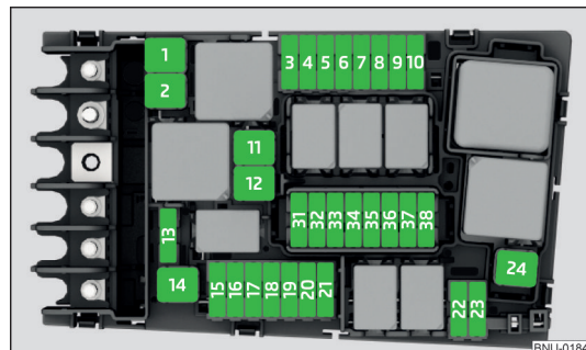
Fig. 345 Fusibles
