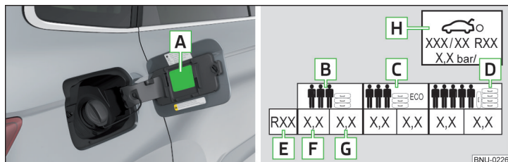
Fig. 312 Adhesivo con una tabla de los valores de presión de llenado de neumáticos / Inflar neumáticos
