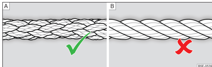
Fig. 327 Cable para remolcar trenzado / Cable para remolcar en espiral
