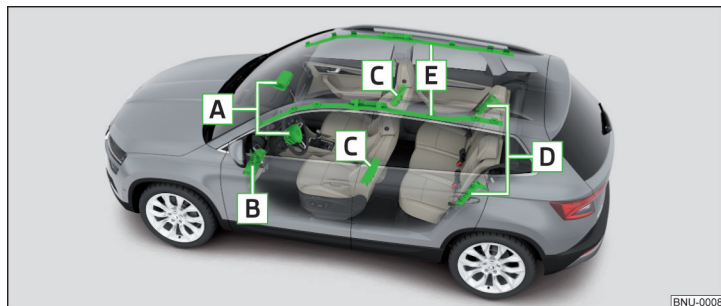
Fig. 21 Lugares de instalación del airbag
