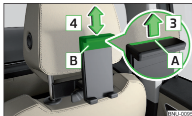
Fig. 136 Ajustar el tamaño del soporte
