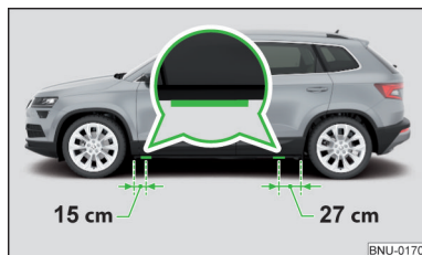
Fig. 323 Travesa de toma para el gato
