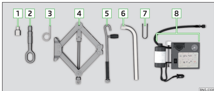
Fig. 317 Equipo de herramientas a bordo
