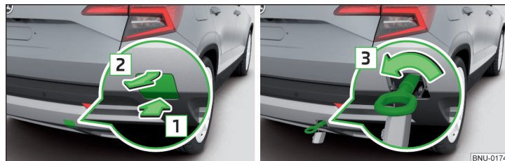
Fig. 329 Retirar la caperuza / instalar la argolla de remolque
