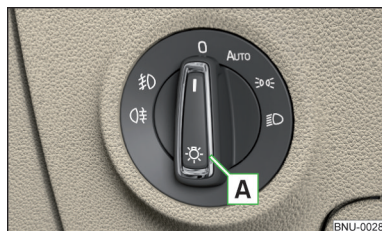
Fig. 62 Conmutador de luces
