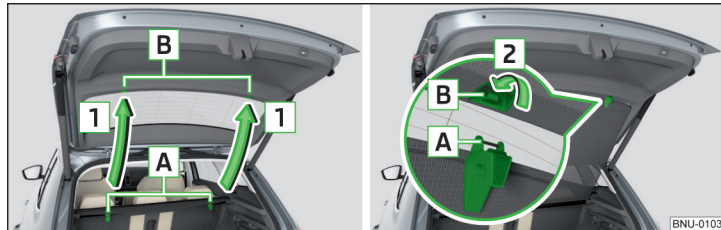
Fig. 146 Fijar la cubierta enrollable en la tapa del maletero
