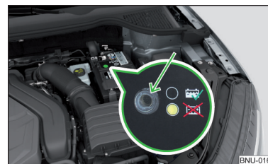
Fig. 311 Batería del vehículo: Indicador del nivel de ácido
