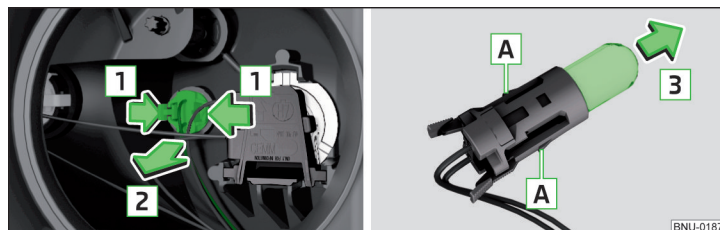
Fig. 348 Cambiar la bombilla de la luz de población
