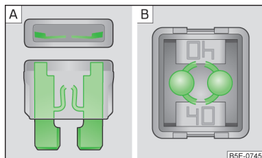
Fig. 340 Fusibles quemados
