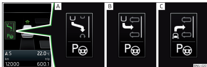
Fig. 273 Menú con los modos de aparcamiento: Visualización en pantalla
