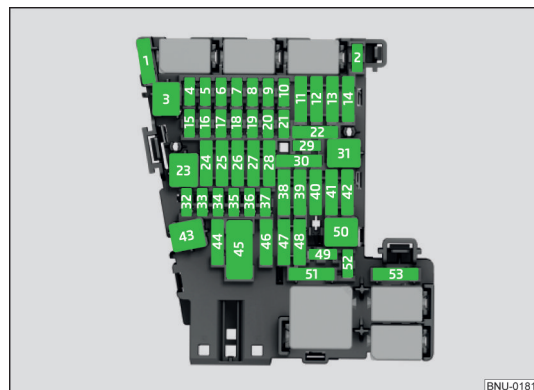
Fig. 343 Fusibles
