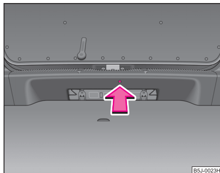
Fig. 26 Desbloqueo de emergencia del portón posterior
