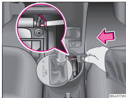
Fig. 109 Desbloqueo de emergencia de la palanca selectora
