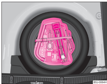
Fig. 166 Maletero: Alojamiento para las herramientas de a bordo
