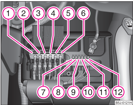
Fig. 182 Representación esquemática de la distribución de fusibles en la batería
