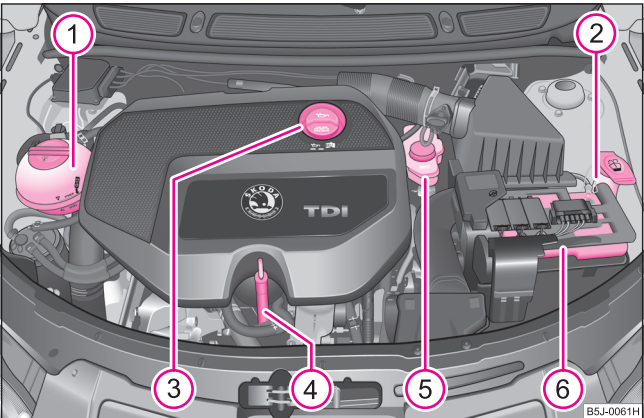
Fig. 156 Motor Diesel de 1,9 l/77 kW
