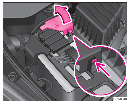
Fig. 160 Batería: Levantar la cubierta
