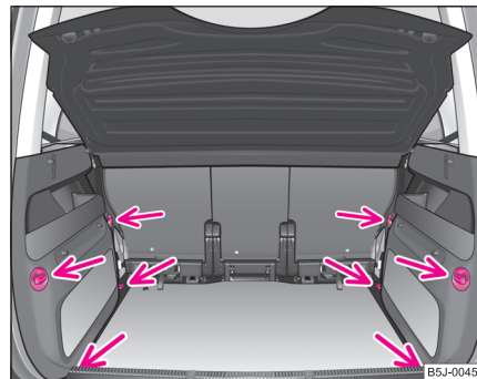
Fig. 60 Maletero: Argollas de amarre y gancho de amarre
