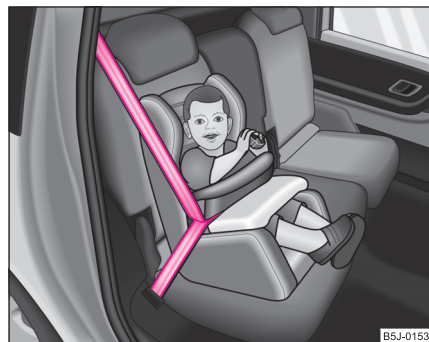
Fig. 139 Asiento infantil instalado en dirección de la marcha con mesa de seguridad del grupo 1 en el asiento trasero
