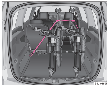
Fig. 71 Fijación de la bicicleta mediante una cuerda
