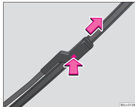
Fig. 43 Escobilla para el parabrisas
