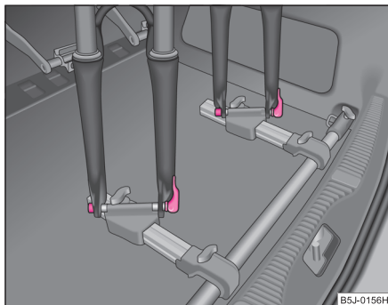
Fig. 68 Poner una bicicleta
