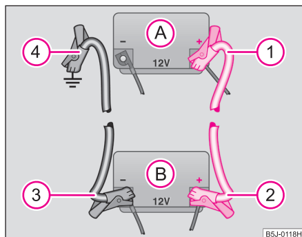
Fig. 174 Ayuda de arranque con la batería de otro vehículo: A - batería descargada del vehículo, B - batería auxiliar
