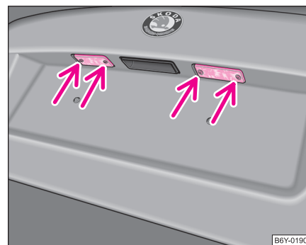
Fig. 189 Desmontar la luz de la matrícula
