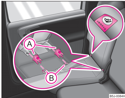
Fig. 142 Argollas de sujeción (sistema ISOFIX)
