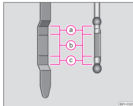
Fig. 157 Varilla de medición de aceite
