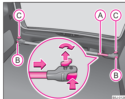
Fig. 66 Montar el travesaño
