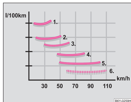
Fig. 148 Consumo de combustible en l/100 km y velocidad en km/h
