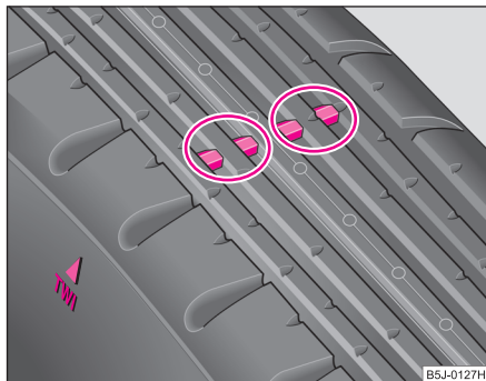
Fig. 164 Perfil de los neumáticos con indicadores de desgaste
