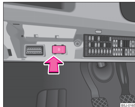
Fig. 33 Cajón de fusibles: Conmutador de la luz de marcha diurna
