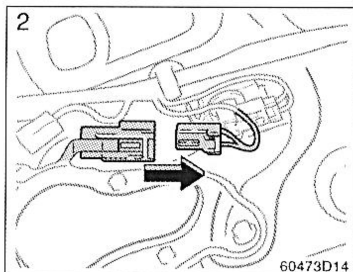
Sólo lado derecho: Después de recambiar la bombilla, enchufe el conector para el motor del limpiavidrios de la ventanilla posterior.
