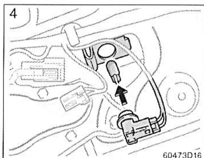
Sólo lado derecho: Desenchufe el conector para el motor del limpiavidrios de la ventanilla posterior.
