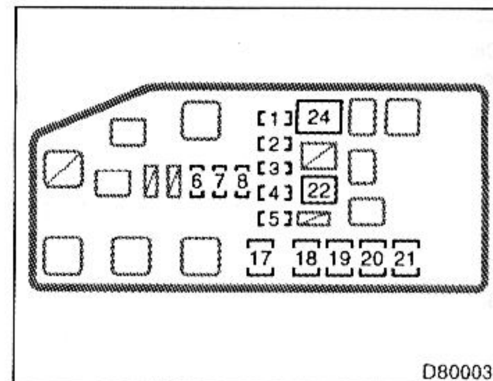
Compartimiento del motor
