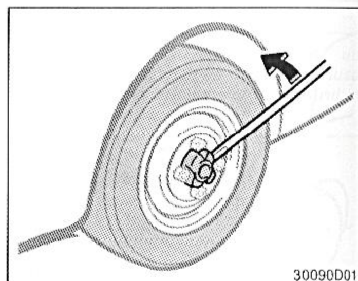
Ruedas de acero (tipo A)
