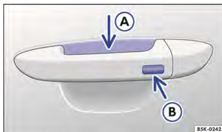
Fig. 55 Sistema de cierre y arranque Keyless Access sin llave: superficie del sensor (A) para desbloqueo en la parte interior de la manilla de la puerta y superficie del sensor (B) para cierre en la parte exterior de la manilla de la puerta.
