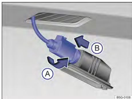
Fig. 136 Luz de la placa de licencia: desinstalar el portalámparas.
