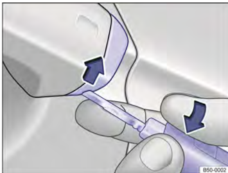
Fig. 58 Manilla de la puerta del conductor: levantar la caperuza.
