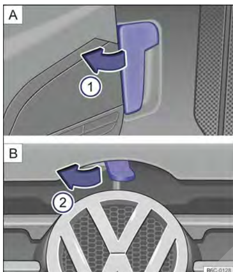
Fig. 145 [A] Palanca de desbloqueo de la tapa del compartimento del motor en la zona reposapiés del conductor. [B] Palanca de desbloqueo en la parte interior de la tapa del compartimento del motor.
