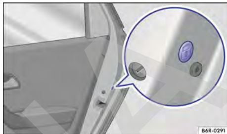
Fig. 59 En la puerta trasera: cierre de emergencia, cubierto por una junta de goma.
