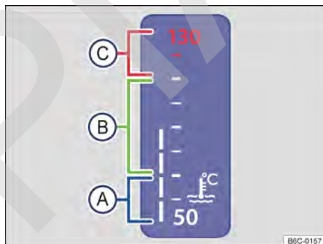
Fig. 18 Indicador de temperatura del líquido de refrigeración del motor en instrumento combinado digital: (A) zona fría; (B) zona normal; (C) zona de alerta.
