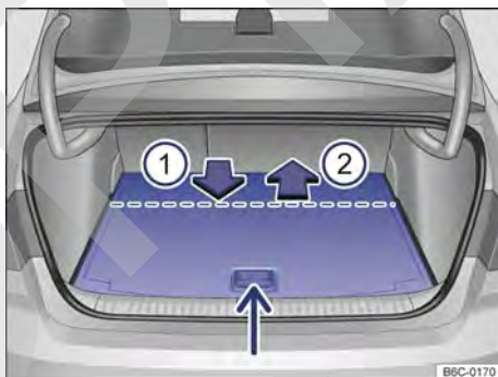
Fig. 115 En el maletero: regular la altura del piso variable del maletero.
