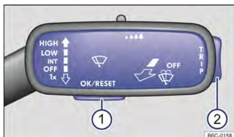
Fig. 21 En vehículos sin volante multifunción: tecla ① en la palanca de los limpiaparabrisas para confirmar los ítems de menú y llave ② para intercambiar entre los menús.
