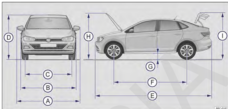
Fig. 174 Dimensiones.
