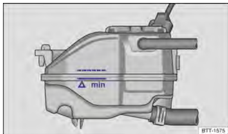
Fig. 151 En el compartimento del motor: marca en el depósito de expansión del líquido refrigerante del motor.
