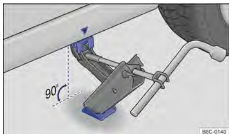
Fig. 167 Puntos de apoyo del gato y gato posicionado atrás en el lado izquierdo trasero del vehículo.
