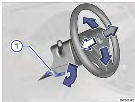
Fig. 64 Debajo y a la izquierda del volante junto con el revestimiento de la columna de dirección: palanca de ajuste de la posición del volante.
