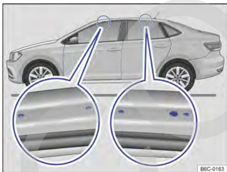
Fig. 118 Puntos de fijación de los soportes básicos del portaequipaje de techo (ambos lados)
