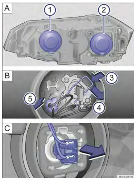
Fig. 127 En el compartimento del motor: ⓘ farol alto y luz de posición y ⓘ farol bajo.
