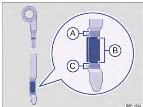
Fig. 149 Varilla de medición del aceite con marca de nivel de aceite del motor.
