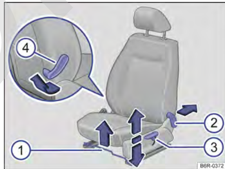
Fig. 66 En el asiento delantero: comandos.
