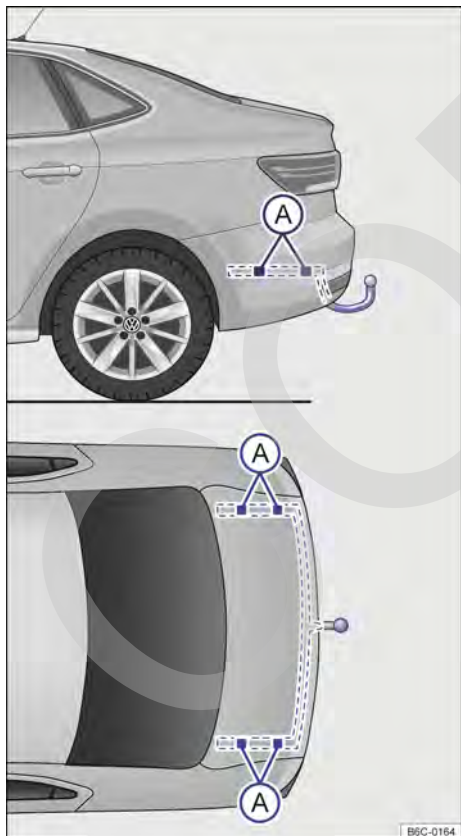
Fig. 119 Puntos de fijación para el montaje posterior de un enganche para remolque.
