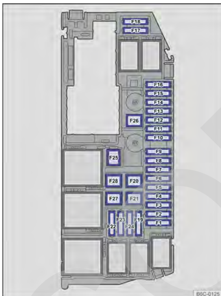
Fig. 140 En el compartimento del motor: disposición de los fusibles.
