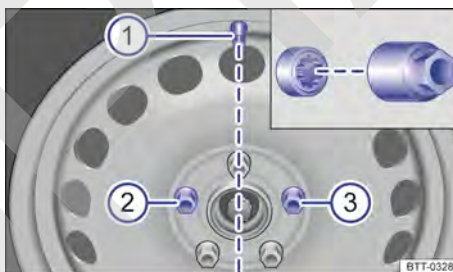
Fig. 165 Cambio de rueda: válvula del neumático ① y posición de montaje del tornillo de la rueda anti-robo ② o ③.
