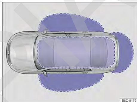
Fig. 54 Sistema de cierre y arranque Keyless Access sin llave:  reas de aproximaci n.
