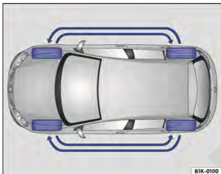
Fig. 156 Esquema para cambio de las ruedas.
