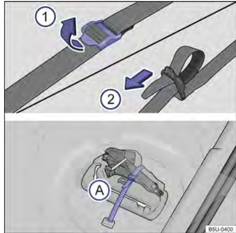
Fig. 122 En el maletero: cinta de fijación de la caja de herramientas y caja de herramientas de a bordo.
