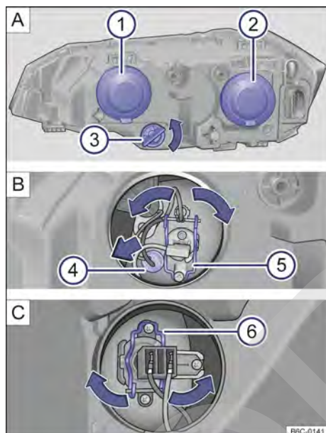
Fig. 129 En el compartimento del motor: ⓘ farol alto y luz de posición, ⓘ farol bajo y ⓘ indicador de dirección.
