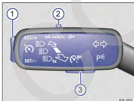
Fig. 98 A la izquierda en la columna de dirección: palanca con interruptor y teclas de mando del GRA.
