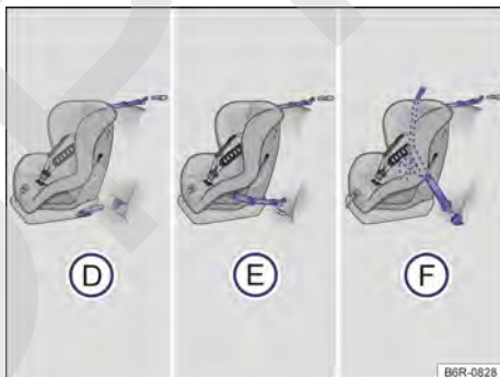
Fig. 43 En el asiento trasero: las figuras D y E muestran el principio de fijación del sistema de retención infantil en los ojales de retención inferiores y con el cinturón de fijación superior. La figura F muestra la fijación del sistema de retención para niños con el cinturón de seguridad del vehículo y con el cinturón de fijación superior.
