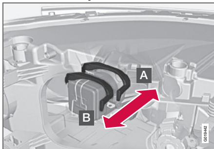
Mando de adaptación del haz luminoso.
