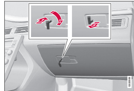
Activación del cierre de privacidad.
