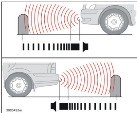
Control de distancia de aparcamiento, parte delantera y parte trasera
