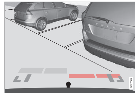
Los campos de colores (uno por sensor) indican la distancia.
