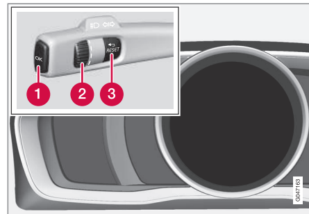
Display y mandos para controlar el menú.
