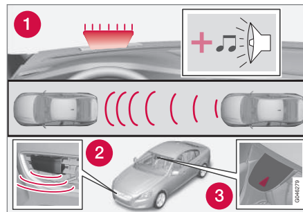
1. Señal acústica y visual cuando hay riesgo de colisión 19 .
