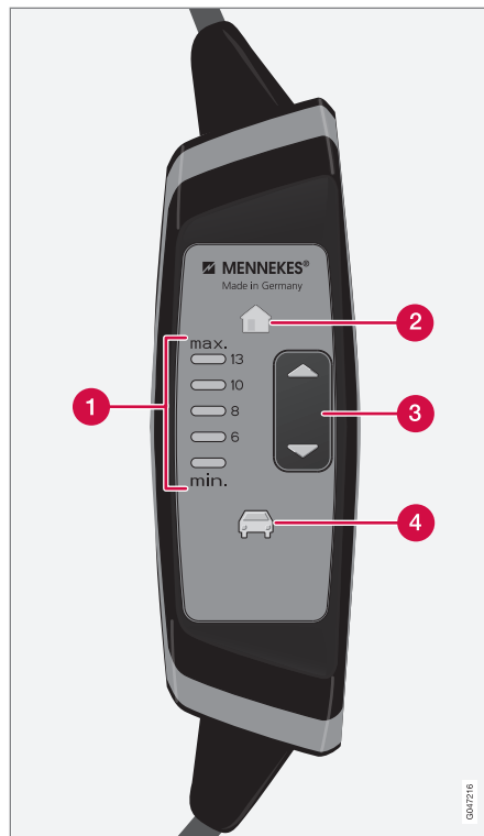
Indicadores e interruptores de la unidad de control.
