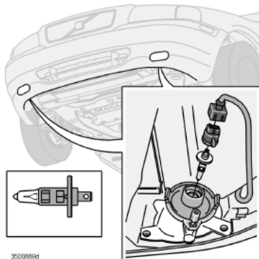
Luces antiniebla
