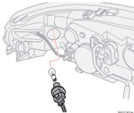
Lámpara de intermitente, lado izquierdo
