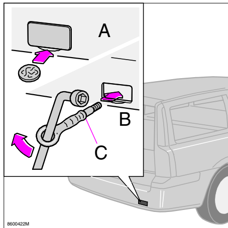
Anilla de remolque trasera
